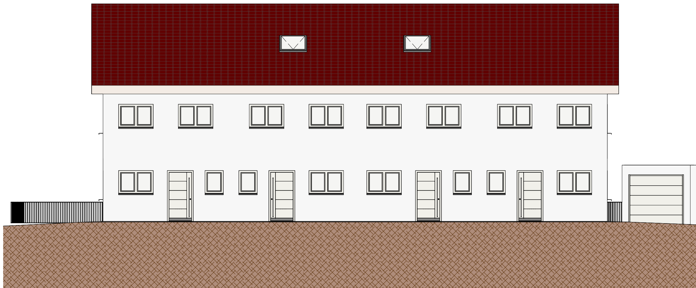
ANSICHT OST
